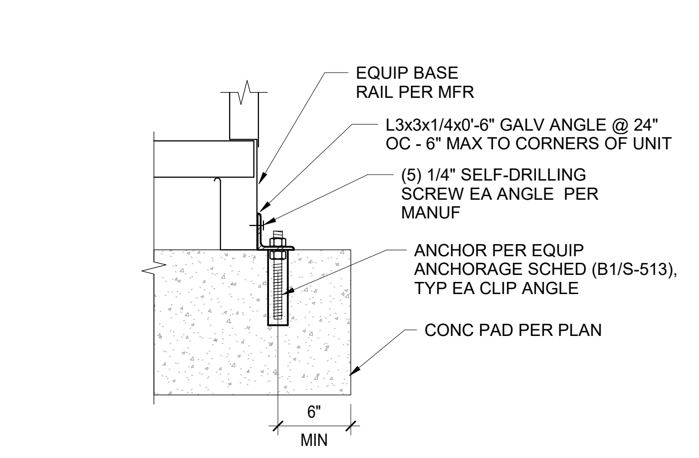
F1 TYP ACU01-A1 ANCHORAGE S-514 SCALE: 1 1/2" = 1'-0"
